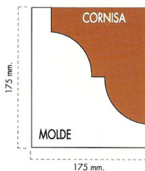
PERFIL 2
