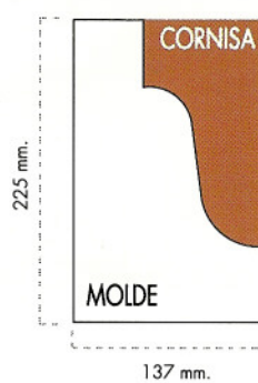
PERFIL 8
