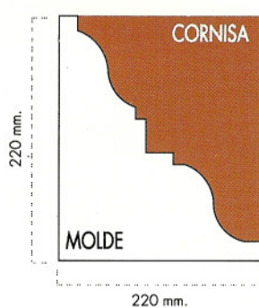
PERFIL 8
