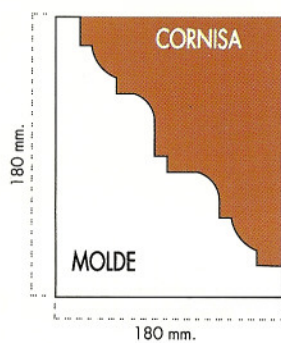
PERFIL 1
