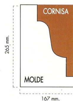
PERFIL 3
