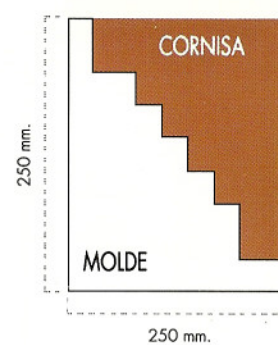
PERFIL 9
