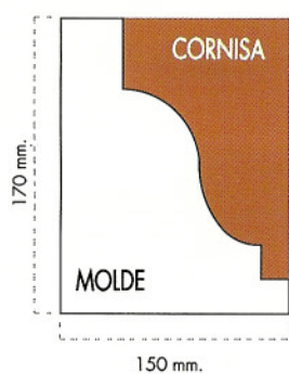
PERFIL 7
