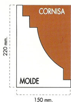
PERFIL 7
